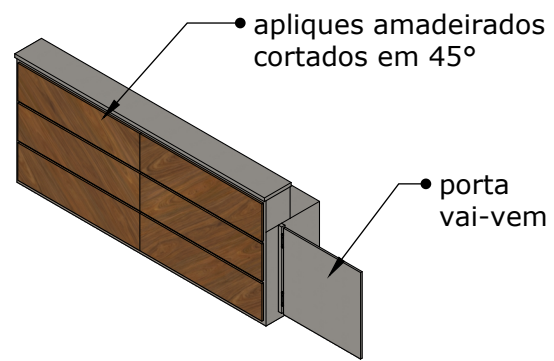
vista perspectiva 1:50
