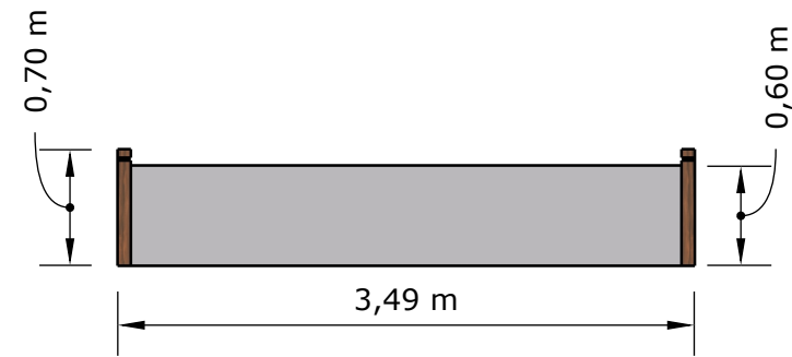
vista topo 1:50
