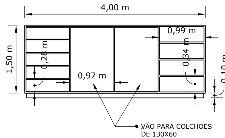
vista frontal interno 1:50
