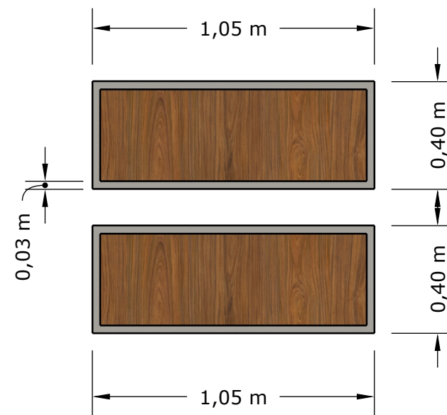
vista frontal 1:20
