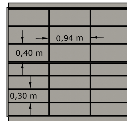
vista frontal (interno) 1:50
