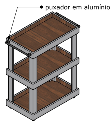
vista perspectiva 1:20
