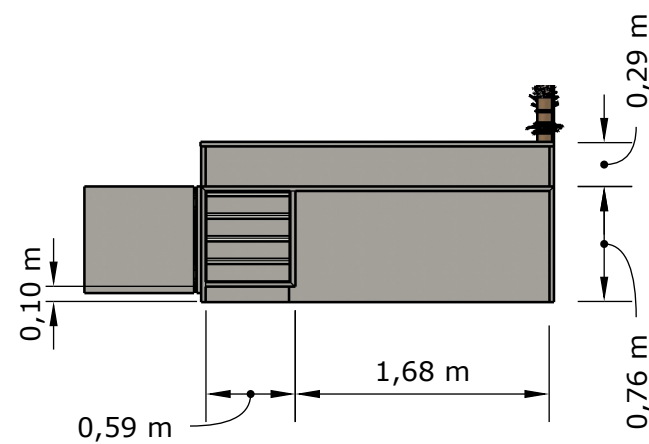
vista frontal (interno) 1:50
