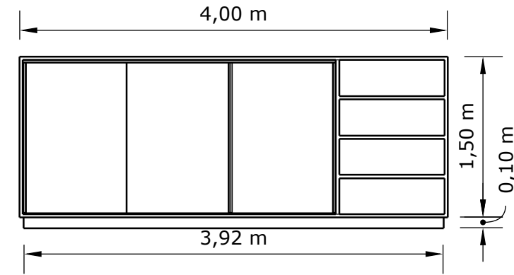
vista frontal externo 1:50
