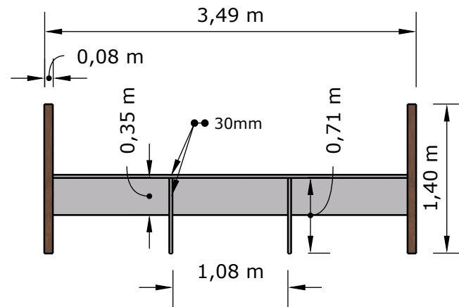
vista frontal 1:50
