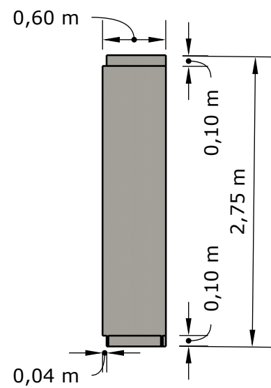
vista lateral 1:50
