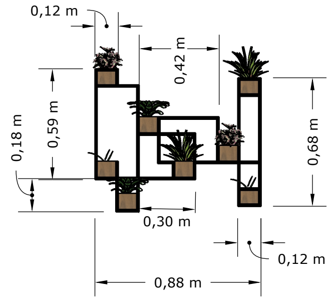
vista frontal 1:20
