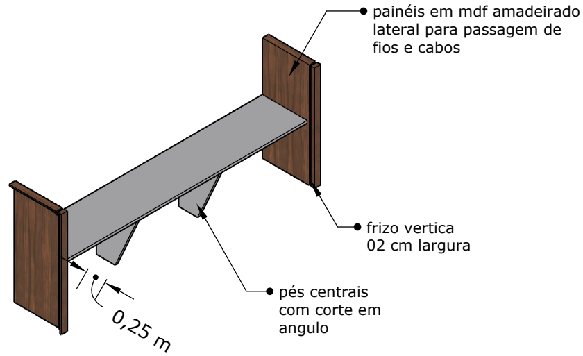
vista perspectiva 1:50
