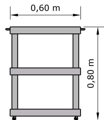
vista frente 1:20
