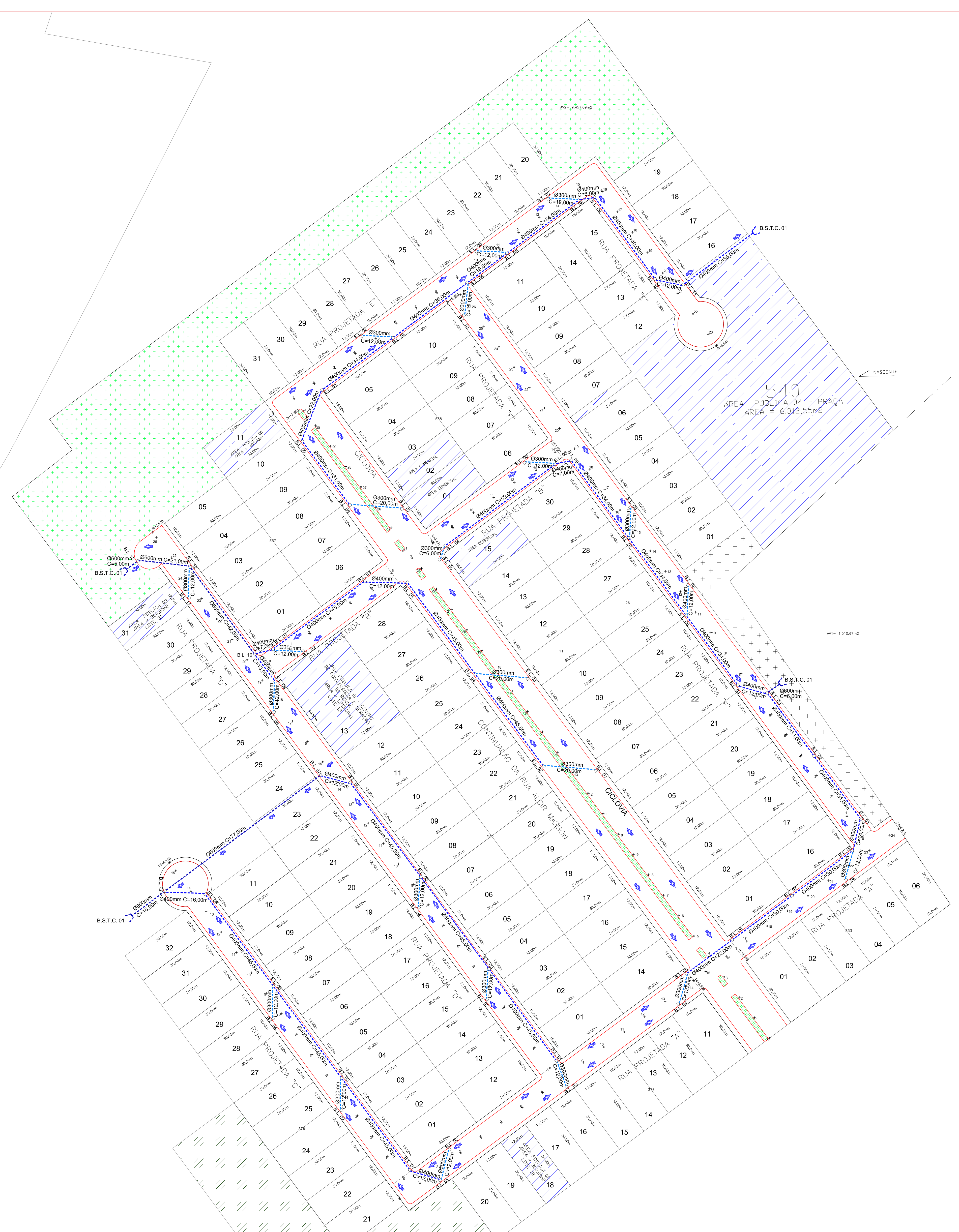
PLANTA DE DRENAEM PLUVIAL ESCALA: 1/750
