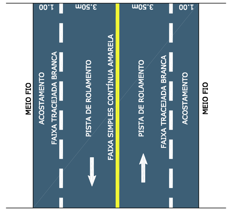
DETALHE DA SINALIZAÇÃO ESCALA: RELATIVA
