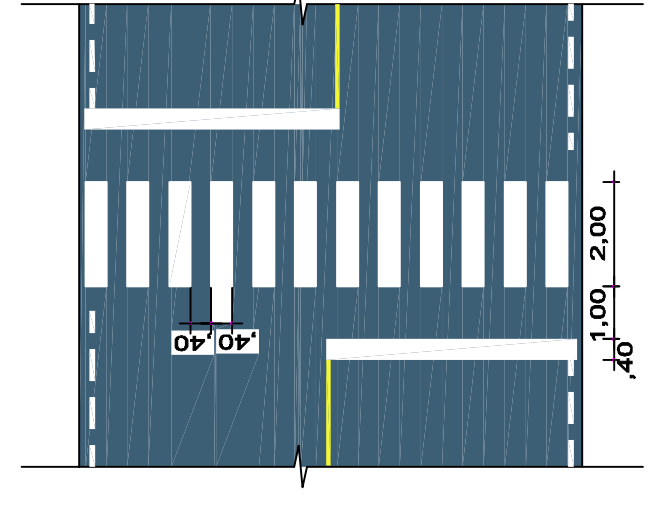
DETALHE FAIXA DE SEGURANÇA P/ PEDESTRES ESCALA: RELATIVA
