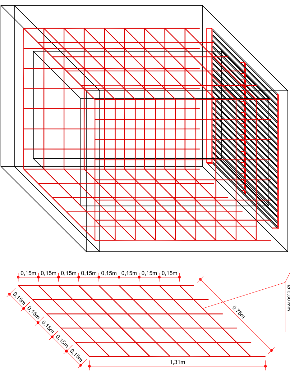
PERSPECTIVA DA CAIXA DE BOCA DE LOBO
