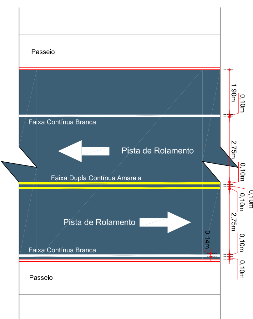
DETALHE DA SINALIZAÇÃO HORIZONTAL ESCALA: 1/100
