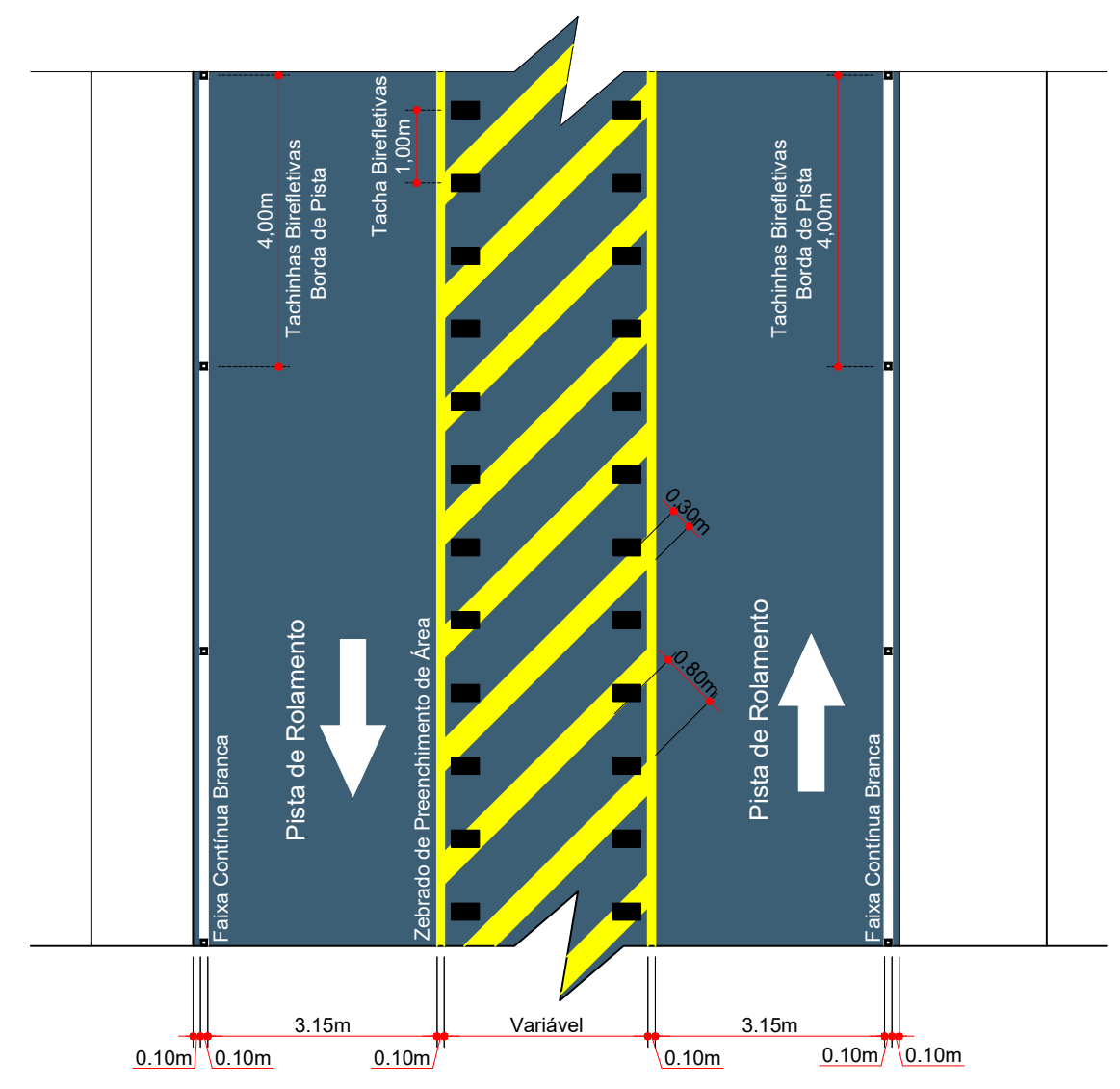
DETALHE DA SINALIZAÇÃO HORIZONTAL ESCALA: 1/100
