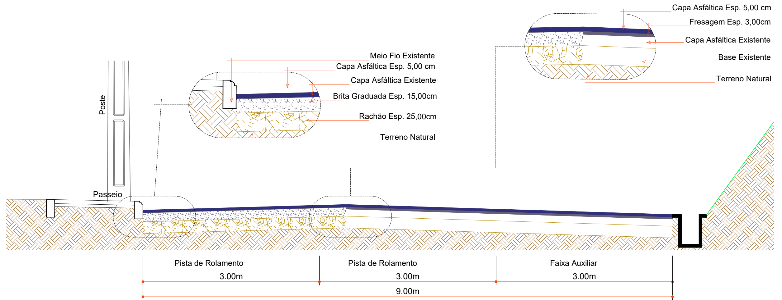
SEÇÃO TRANSVERSAL ESCALA: 1/40 Pavimentação com base nova
