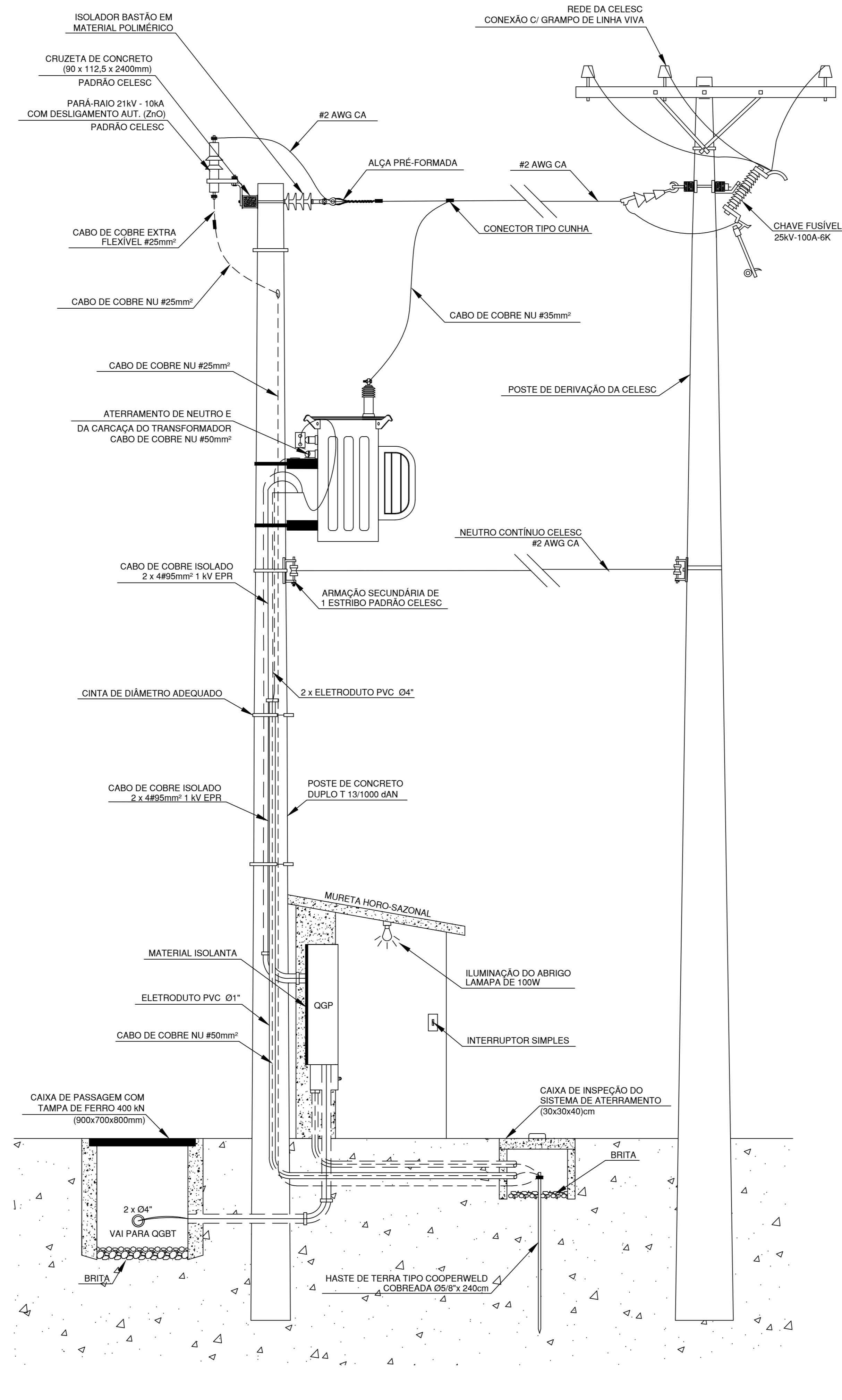
VISTA CORTE LATERAL: A-A" MEDIDAS EM: cm SEM ESCALA
