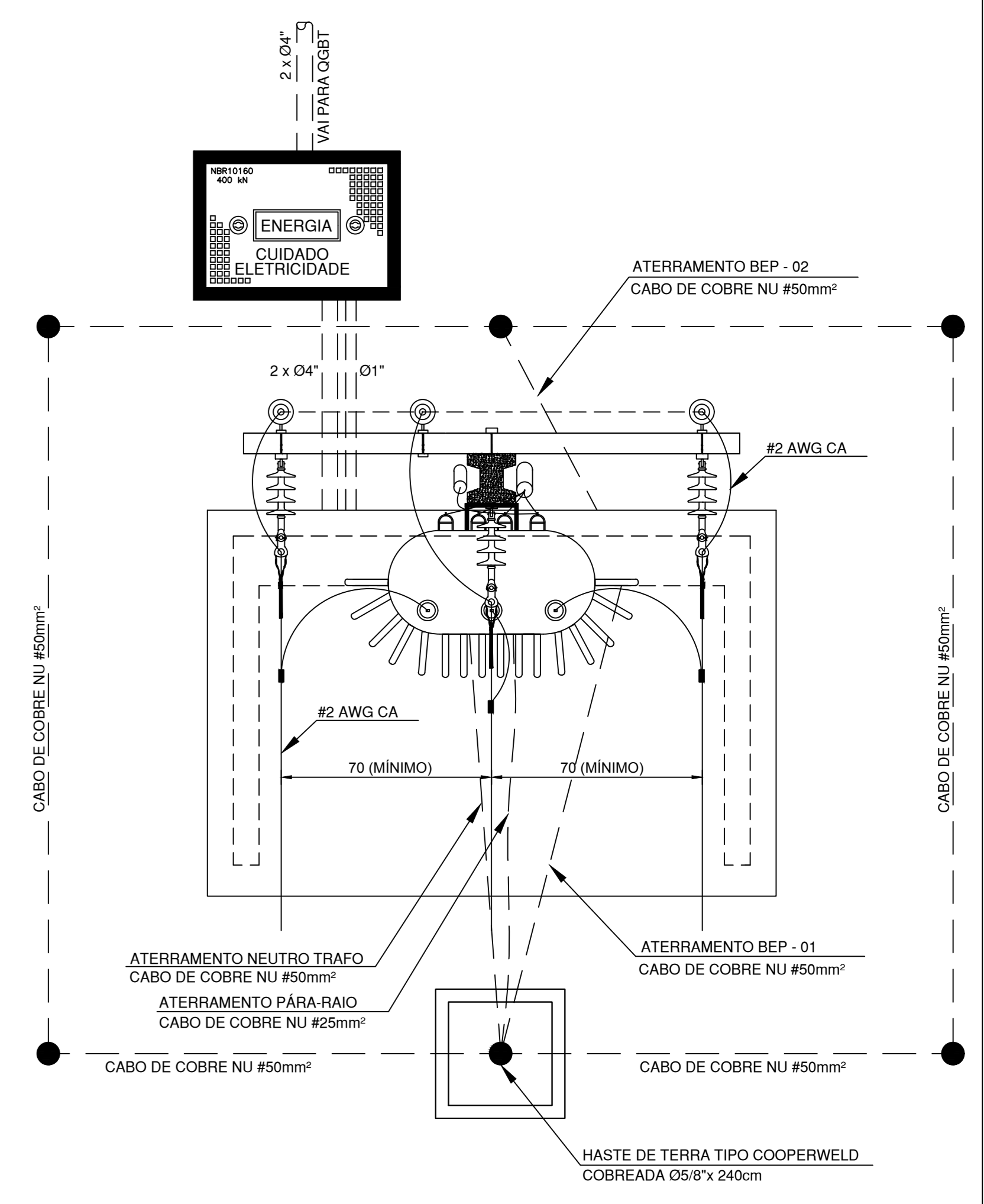
VISTA SUPERIOR MEDIDAS EM: cm SEM ESCALA
