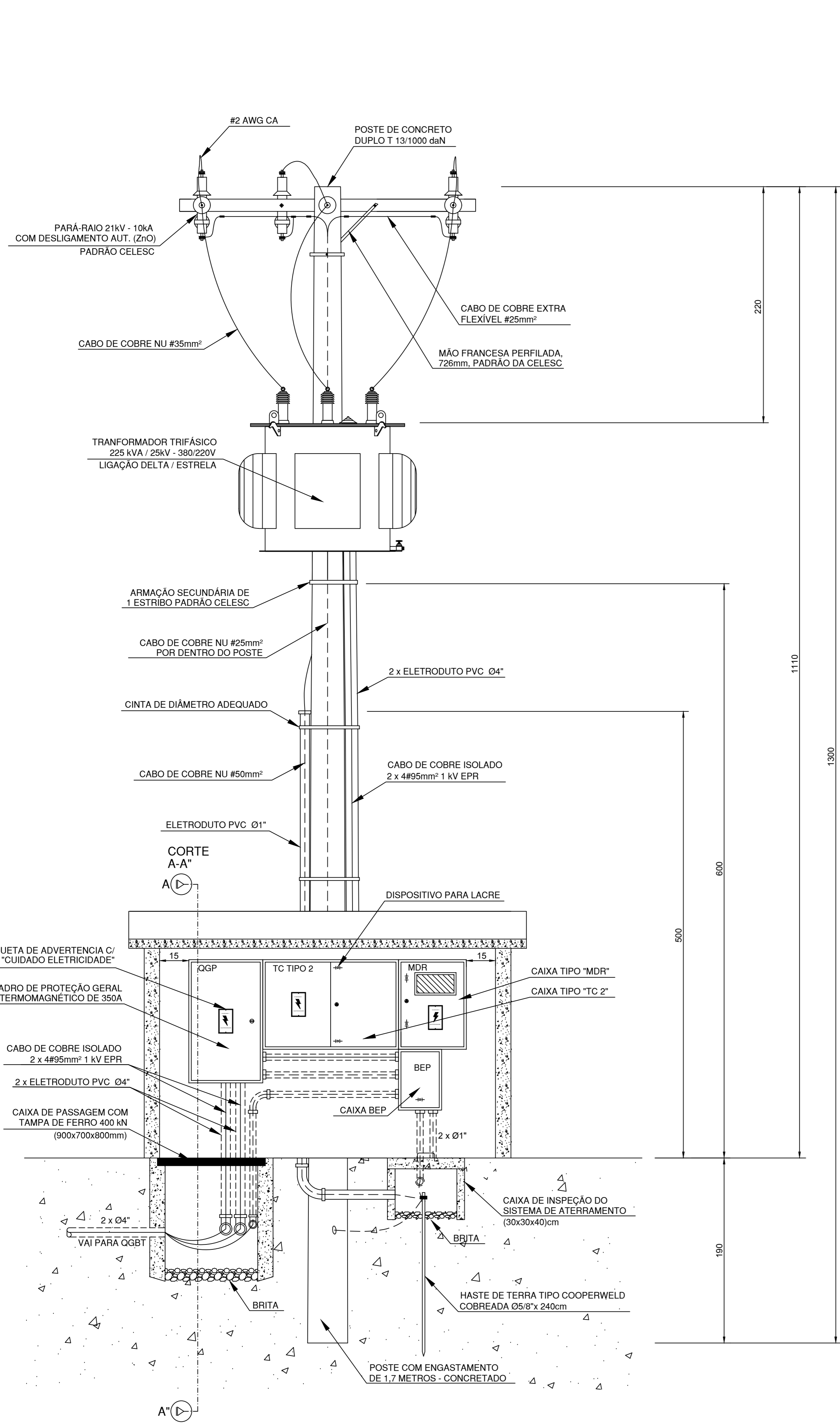
VISTA FRONTAL MEDIDAS EM: cm SEM ESCALA
