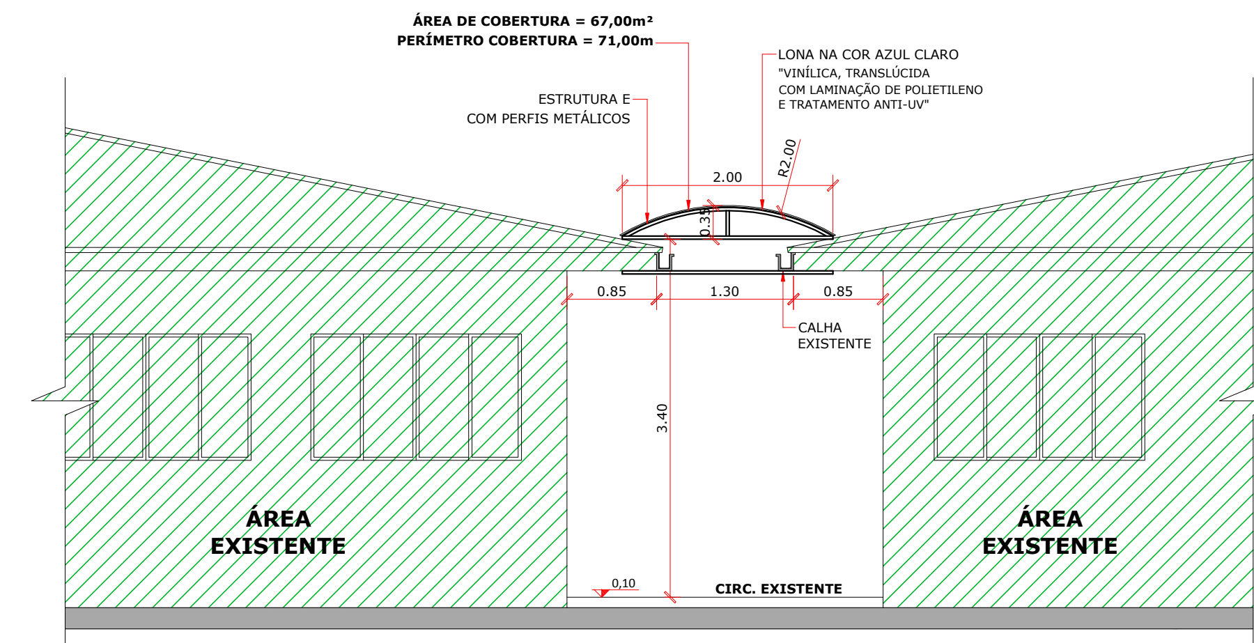
DETALHE CORTE CC ESCALA = 1 : 50
