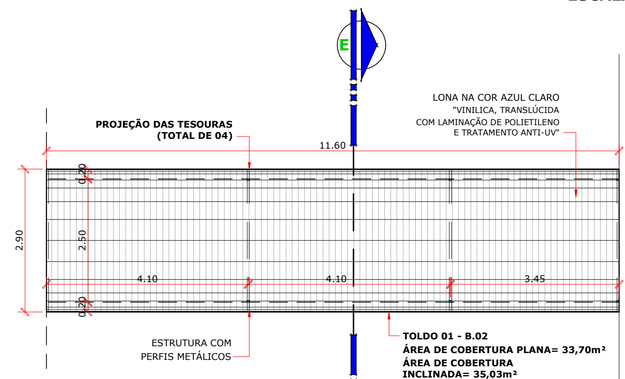
PLANTA DE COBERTURA TOLDO 01 ESCALA = 1 : 75
