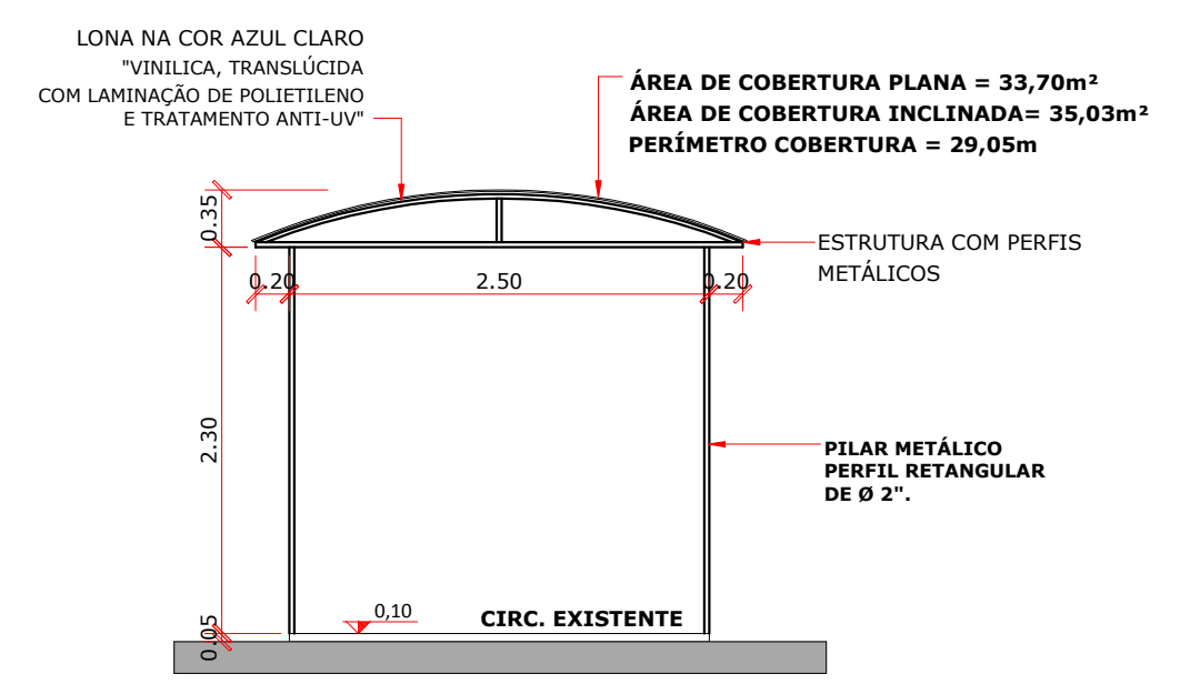
CORTE EE TOLDO 01 ESCALA = 1 : 50
