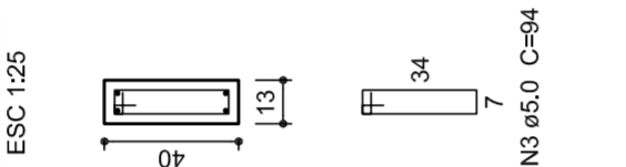
V81 ESC: 1:25
