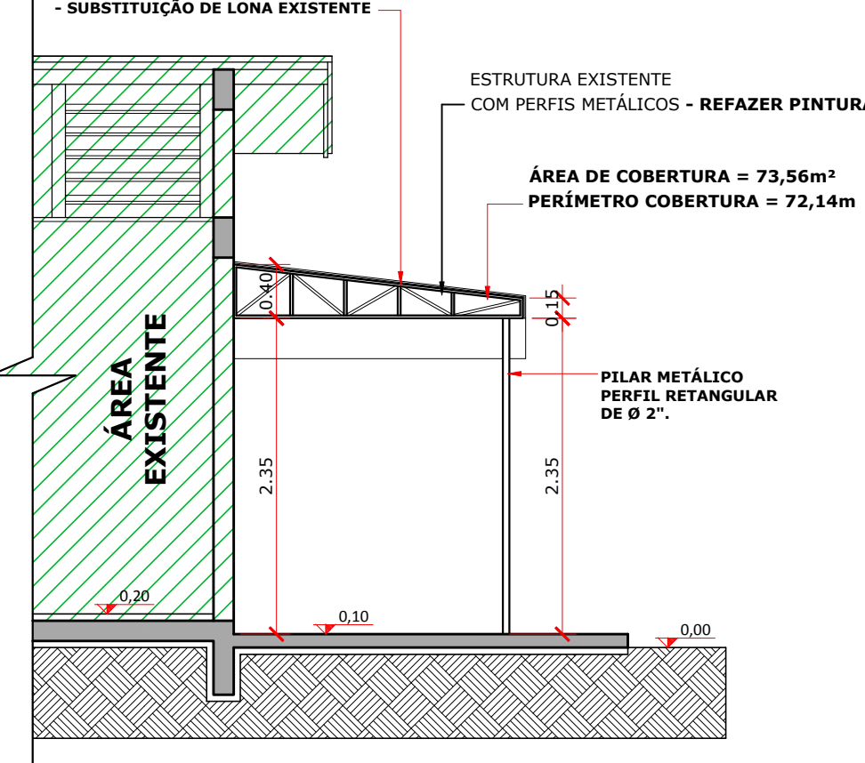
CORTE CC TOLDO 02 - B.01 ESCALA = 1 : 50
