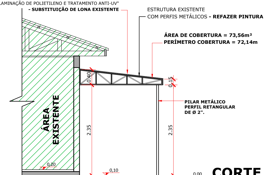
CORTE BB TOLDO 02 - B.01 ESCALA = 1 : 50
